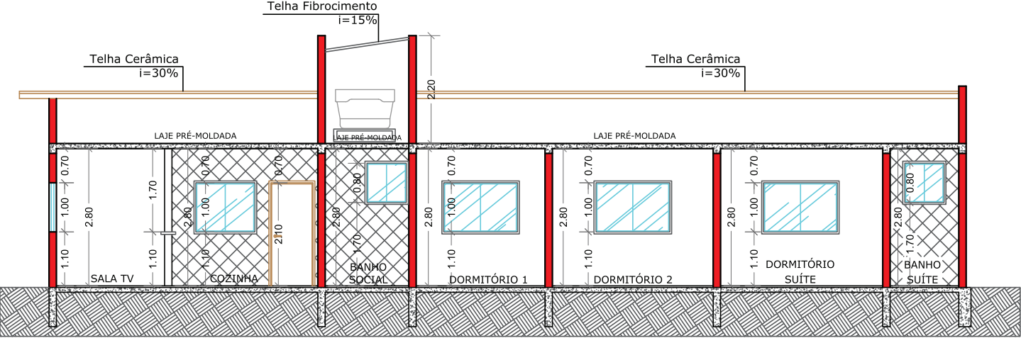
CORTE AA
