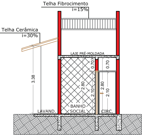
CORTE BB
